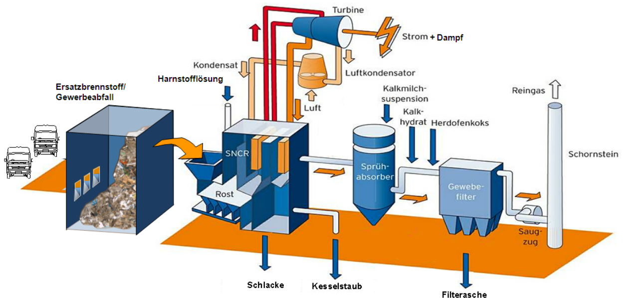
Abbildung 1: Vereinfachtes Verfahrensfliessbild
